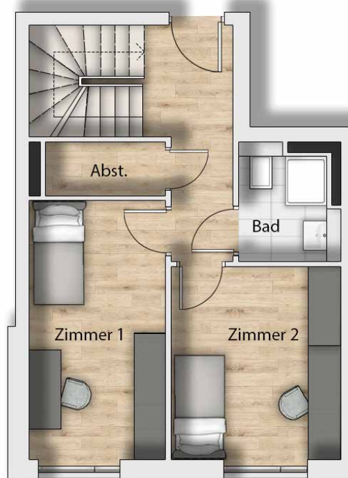
Haus 02 2. OG
